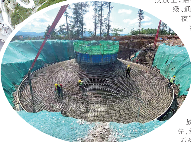
凤凰县两林、禾库风电场建设现场施工图。
