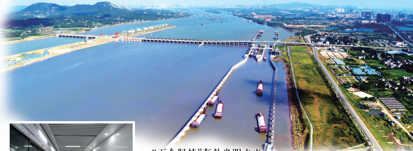
长沙湘江航电枢纽工程
