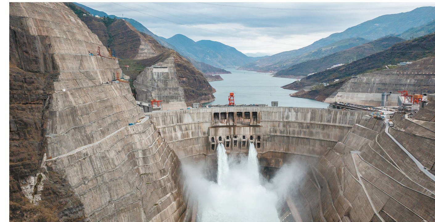
5月20日，位于白鹤滩水电站右岸地下厂房内的9号机组总装工作完成，标志着白鹤滩水电站机组总装工作全部完成，进入全面投产冲刺阶段。白鹤滩水电站位于四川省宁南县和云南省巧家县交界处金沙江干流河段上，是实施“西电东送”的国家重大工程，总装机容量1600万千瓦。 新华社 发
