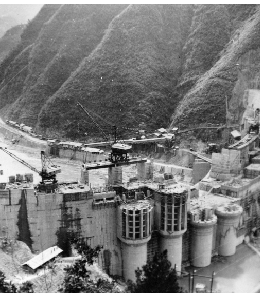
1976年，凤滩水电站大坝施工场景。
